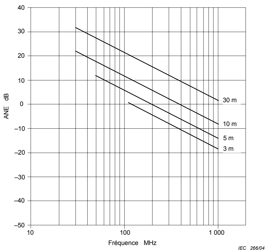
Figure 7 – Graphique de l' ANE théorique en espace libre en fonction de la fréquence pour différentes distances de mesure (voir Equation 4)
