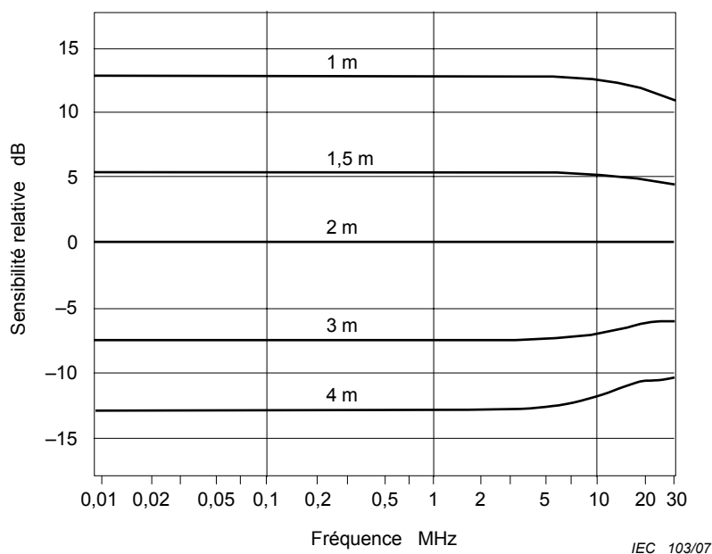
Figure C.11 – Sensibilité S_D d'une antenne cadre de diamètre D par rapport à une antenne cadre de 2 m de diamètre
