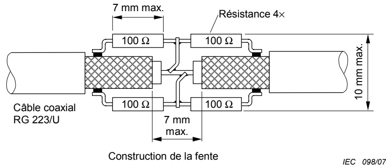
Figure C.3 – Construction de la fente d'une antenne
