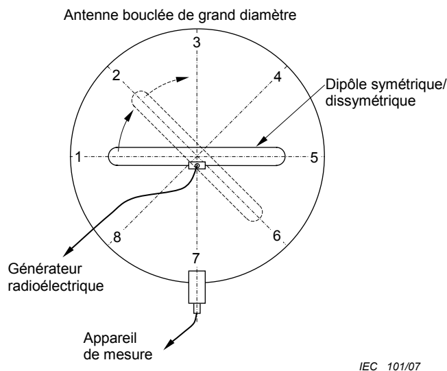
Figure C.7 – Les huit positions du dipôle symétrique/dissymétrique pendant la validation de l'antenne cadre de grand diamètre
