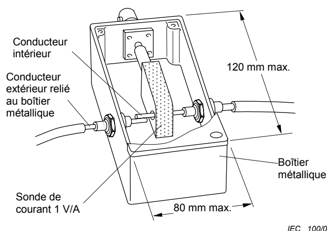
Figure C.5 – Construction du boîtier métallique renfermant la sonde de courant
