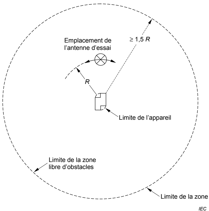
Figure 3 – Zone libre d'obstacles avec appareil en essai fixe (voir 5.3)
