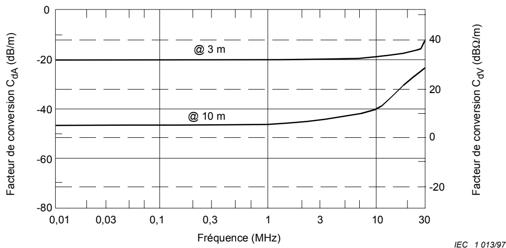
Figure C.10 – Facteurs de conversion C_{dA} (pour la conversion en dB ( \mu A/m )) et C_{dV} (pour la conversion en dB ( \mu V/m )) pour les deux distances de mesure normalisées d
