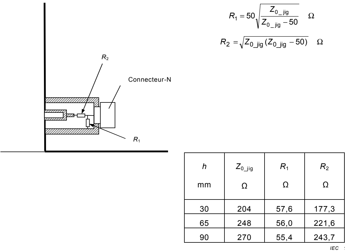
Figure 24 – Exemple d'un adaptateur d'impédance avec réseau résistif
