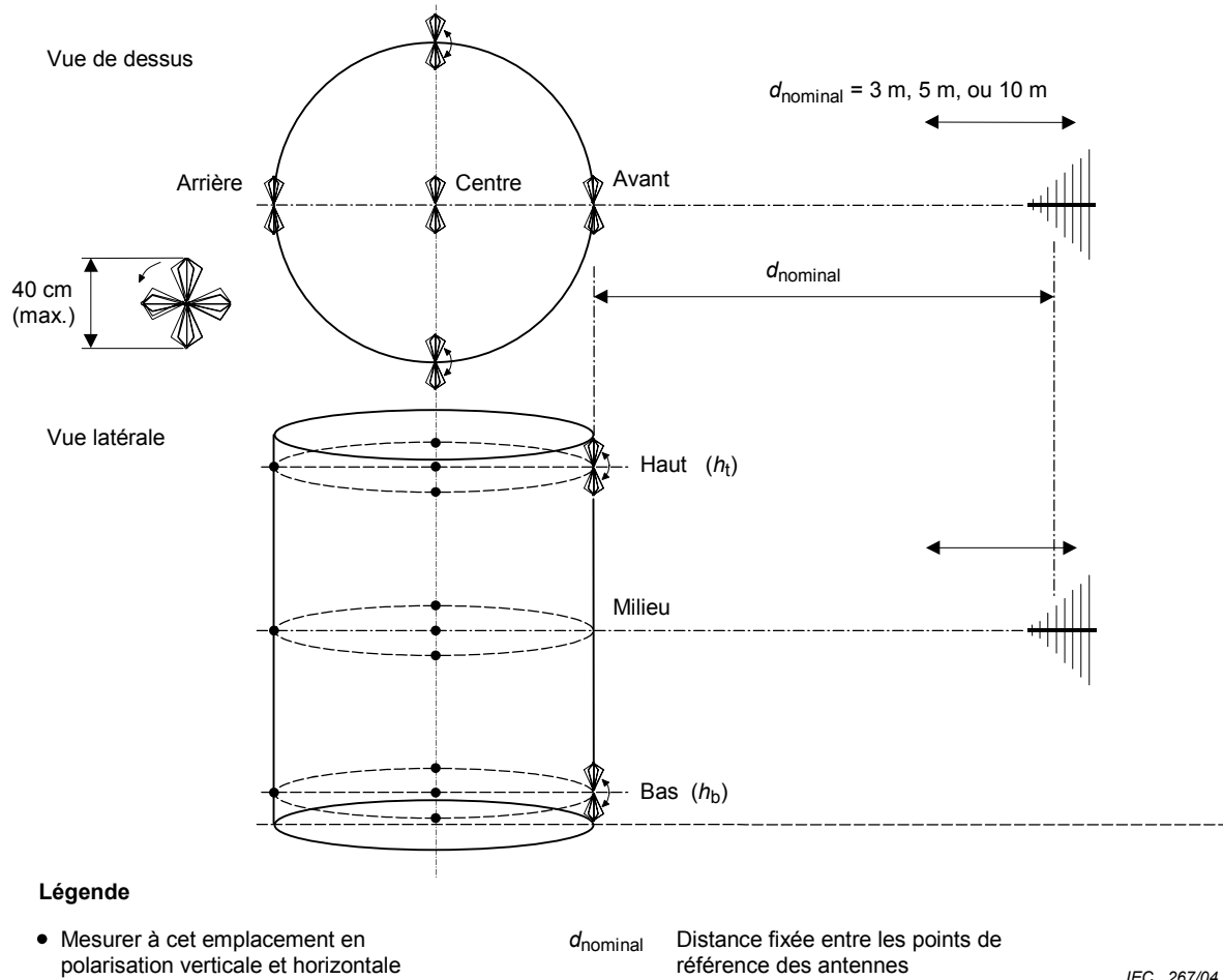
Figure 8 – Positions de mesure pour la procédure de validation de l'emplacement
