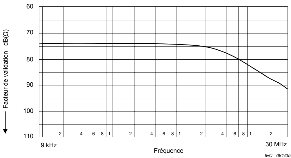
Figure C.8 – Facteur de validation d'une antenne cadre de 2 m de diamètre
