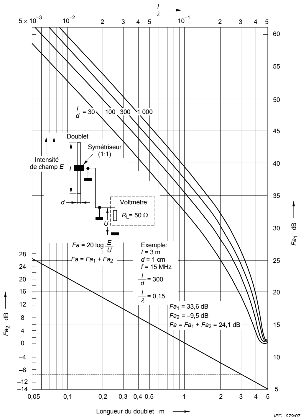
Figure A.1 – Facteurs d'antenne des doublets courts pour R_L = 50 \Omega (voir A.3.2.d) Note)
