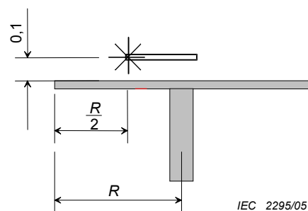
Figure 12 – Position de l'antenne au-dessus de la table d'essai (vue de côté)
