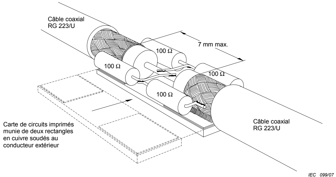
Figure C.4 – Exemple de construction de fente dont la rigidité est assurée par une plaquette de circuit imprimé
