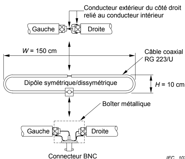
Figure C.9 – Construction du dipôle symétrique/dissymétrique
