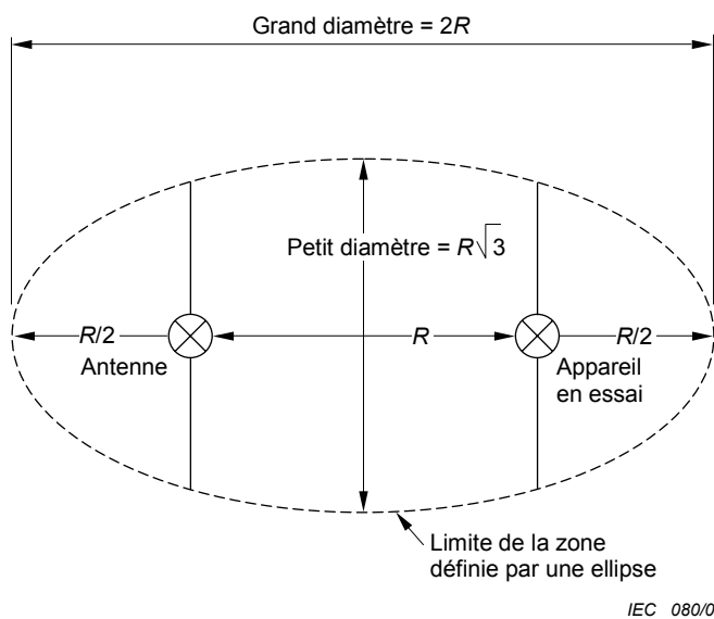
Figure 2 – Zone libre d'obstacles d'un emplacement d'essai équipé d'une table tournante (voir 5.3)
