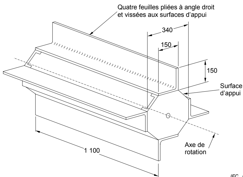
Figure 13 – Exemple d'agitateur typique à aubes
