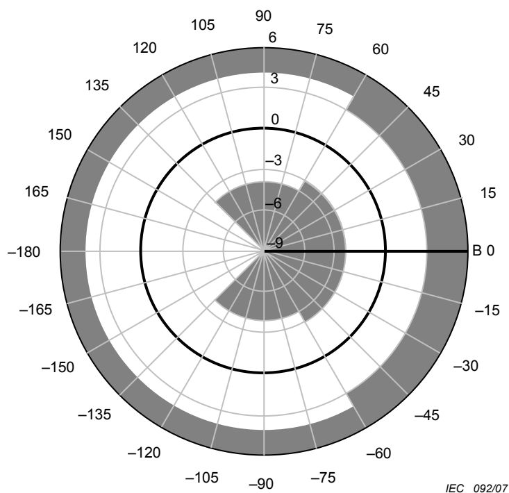
Figure 16b – 6 GHz à 18 GHz
