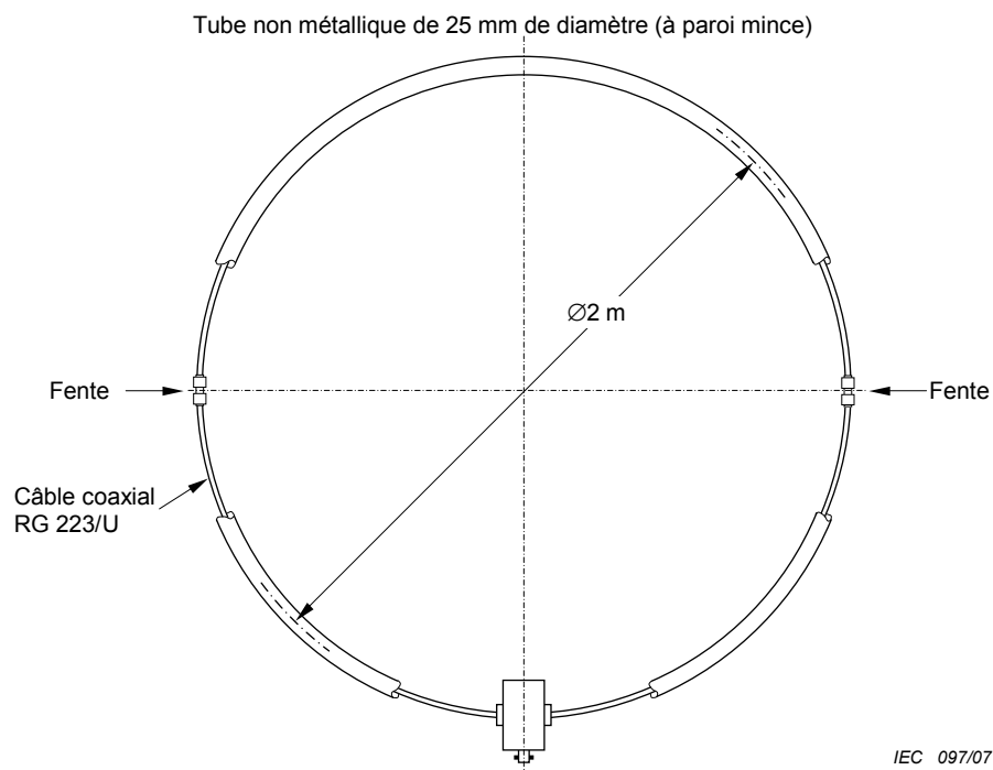
Figure C.2 – Une antenne de grand diamètre, comportant deux fentes diamétralement opposées, placées à égale distance de la sonde de courant C
